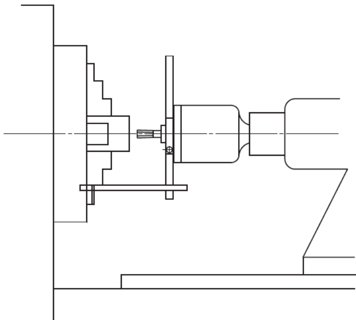
旋盤取付の場合
